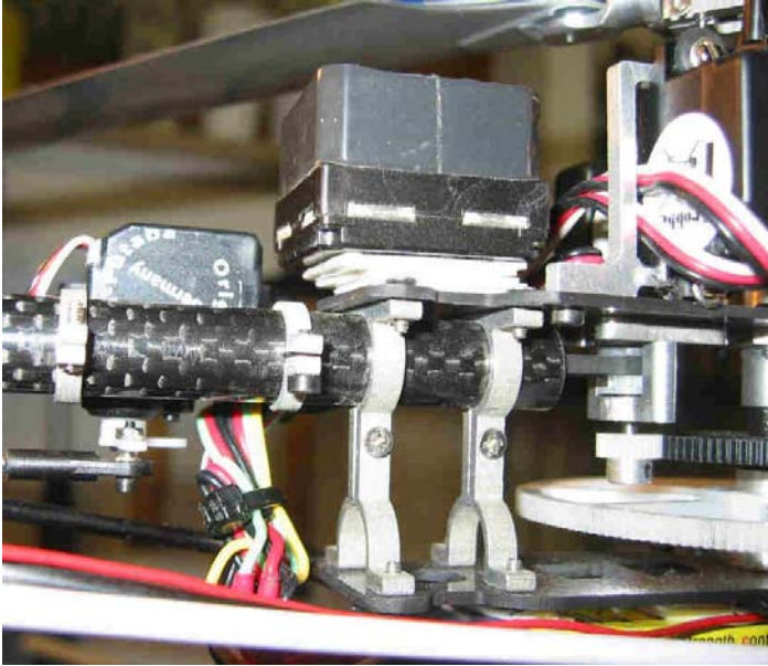
Kreisel GY-401 Unzureichende, weiche Kreiselmontage mit Sechs Lagen Spiegelband (Doppelklebeband)
