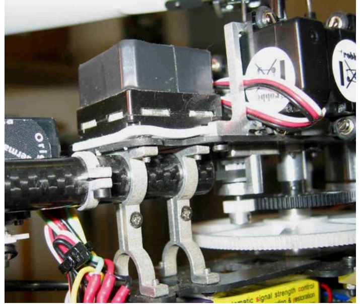
Kreisel GY-401 Zweckmäßige Kreiselmontage mit z.B. Conrad-Servo-Klebeband
